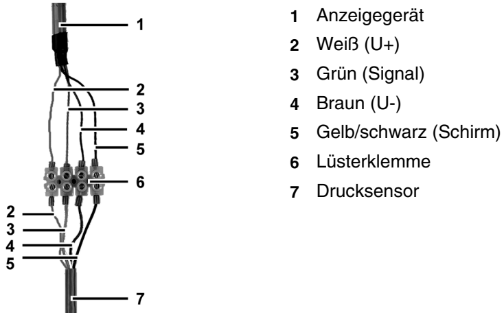
Bild 3: Kabelverbindung
